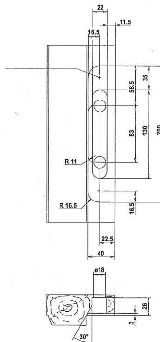
Urtagsritning slutbleck 1887-2
